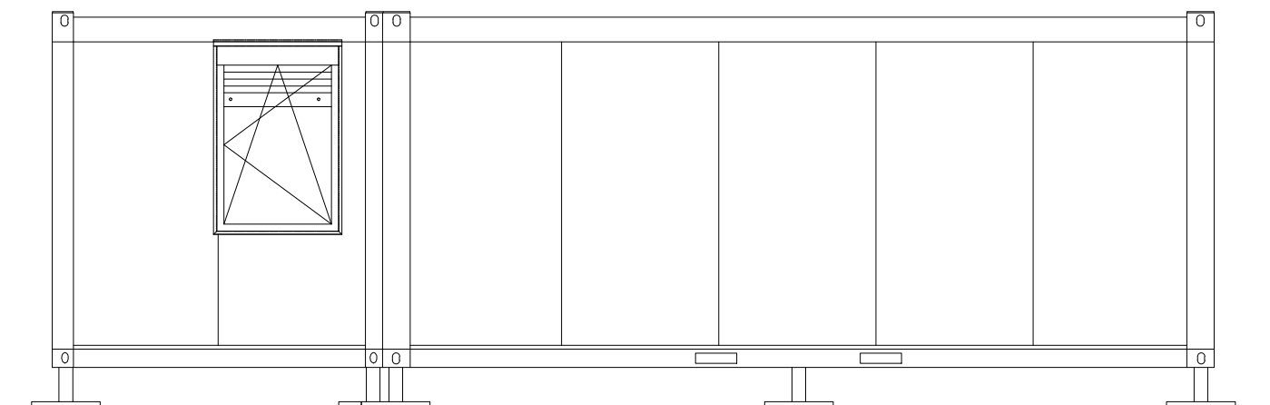
SJEVEROISTOČNO PROČELJE
