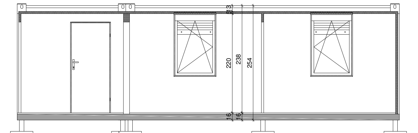
PRESJEK B - B
