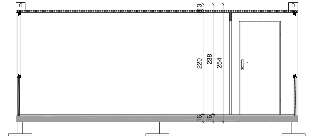
PRESJEK A - A
